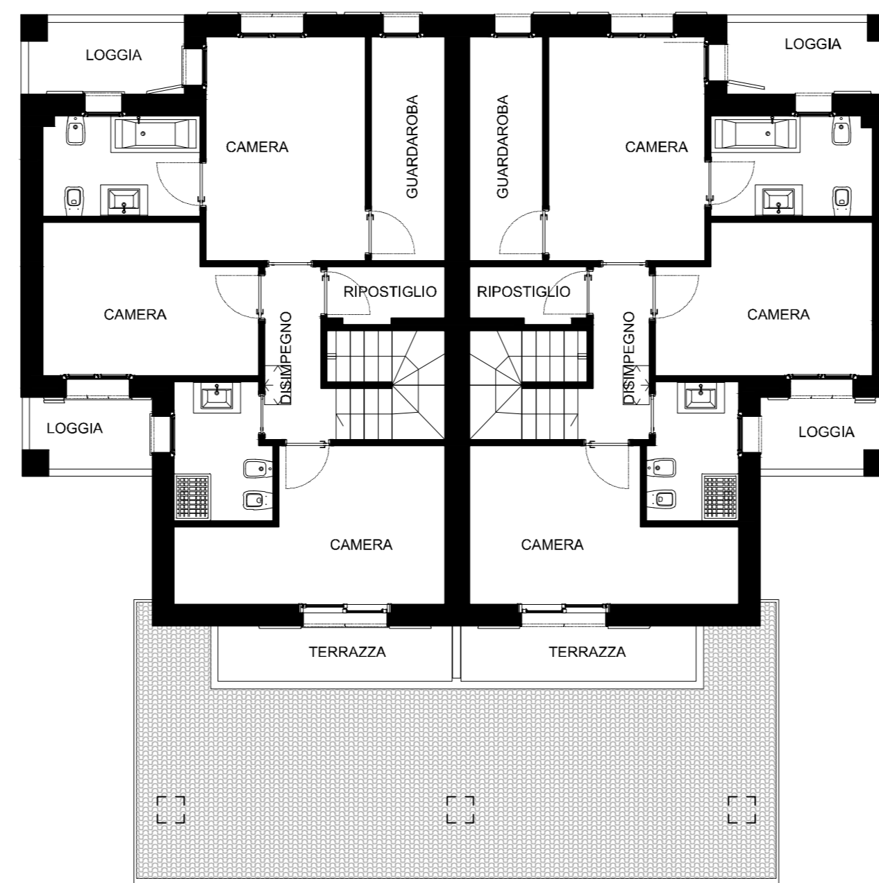
PIANO PRIMO
